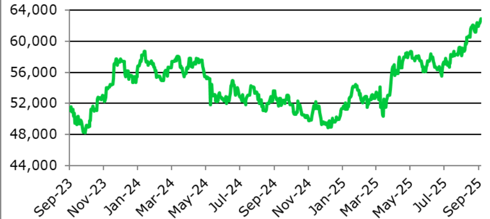
IPC
