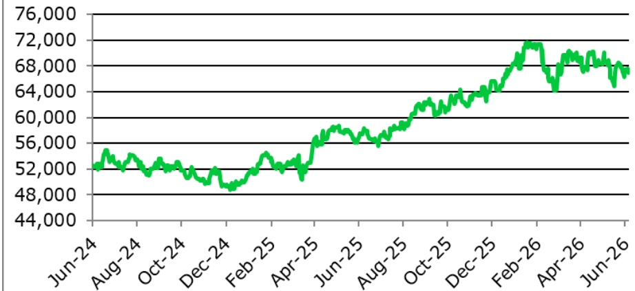
IPC
