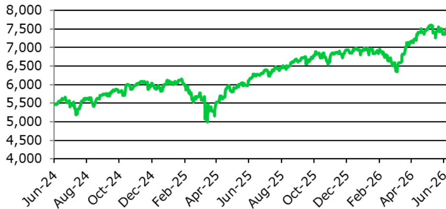
S&P500
